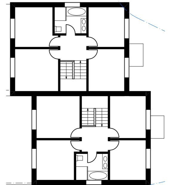
Grundriss Obergeschoss 1 : 200
